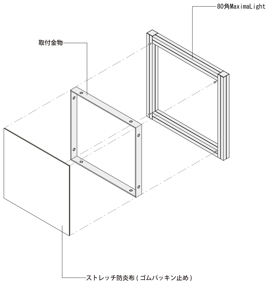
□ファブリックボックス取り付け詳細図
